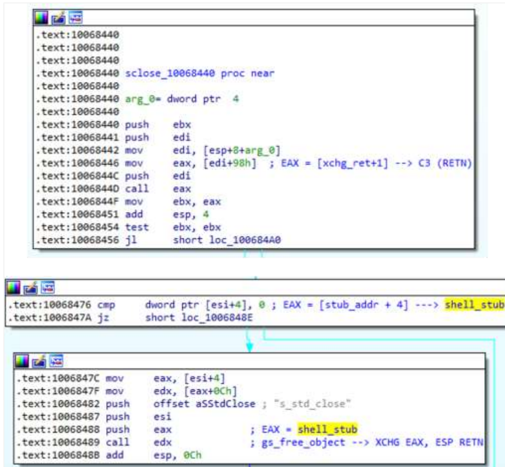
[그림 42] sclose 함수에서 변경된 코드 호출
