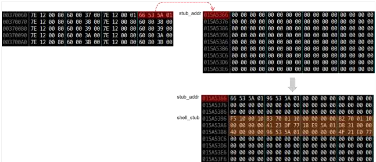
[그림 40] stub_addr +0x30 위치에 shell_stub 생성
