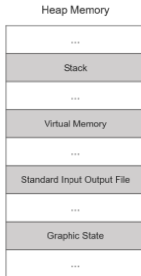
[그림 27] 포스트스크립트 파일 실행을 관리하기 위한 컨텍스트 정보
