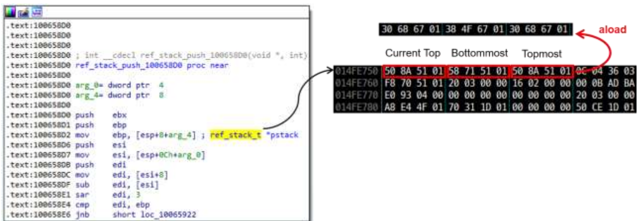
[그림 32] 스택을 초과하는 크기의 배열 로드 시 스택 정보 변경
