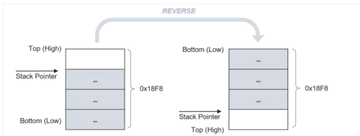
[그림 29] 스택의 모습
