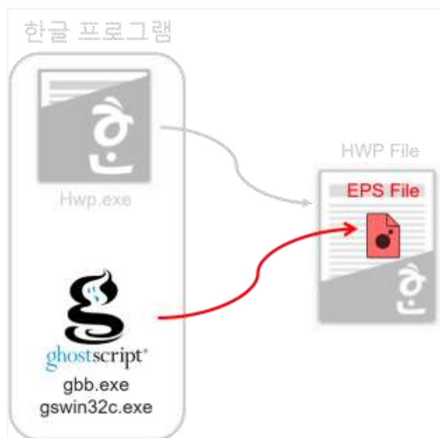
[그림 10] 고스트스크립트의 한글 문서 내 EPS 파일 실행 개념도
