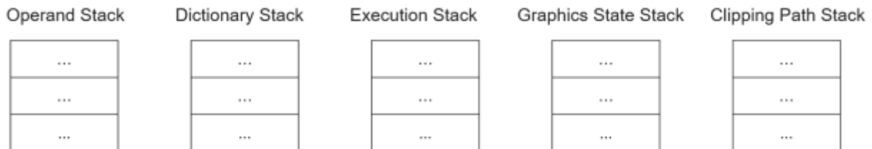
[그림 18] 포스트스크립트 인터프리터가 관리하는 스택
