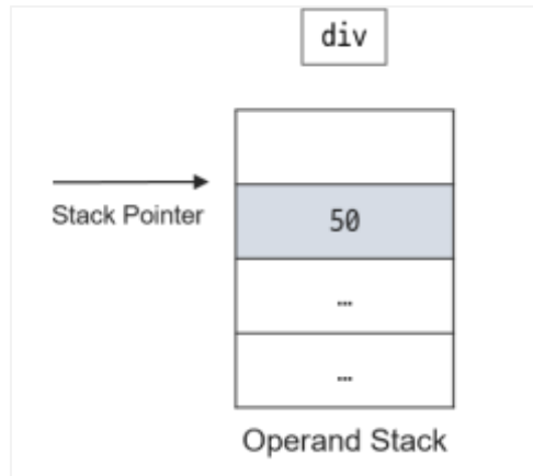
[그림 22] 피연산자 스택
