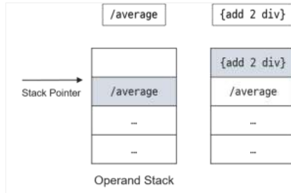
[그림 24] 피연산자 스택
