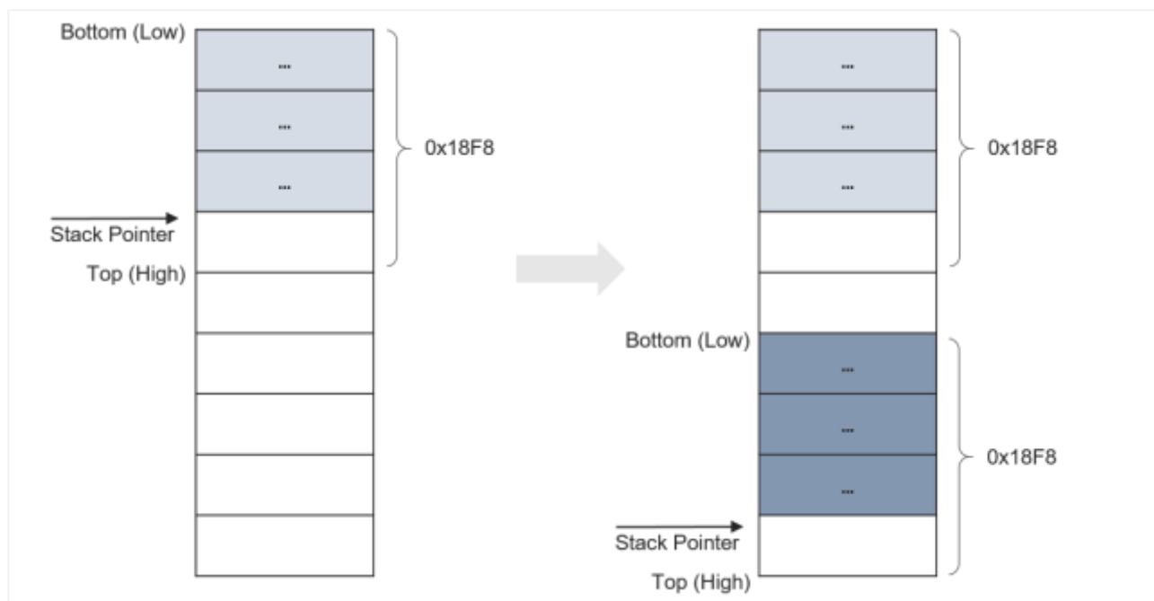
[그림 30] 새로운 스택 할당으로 포인터 주소 증가
