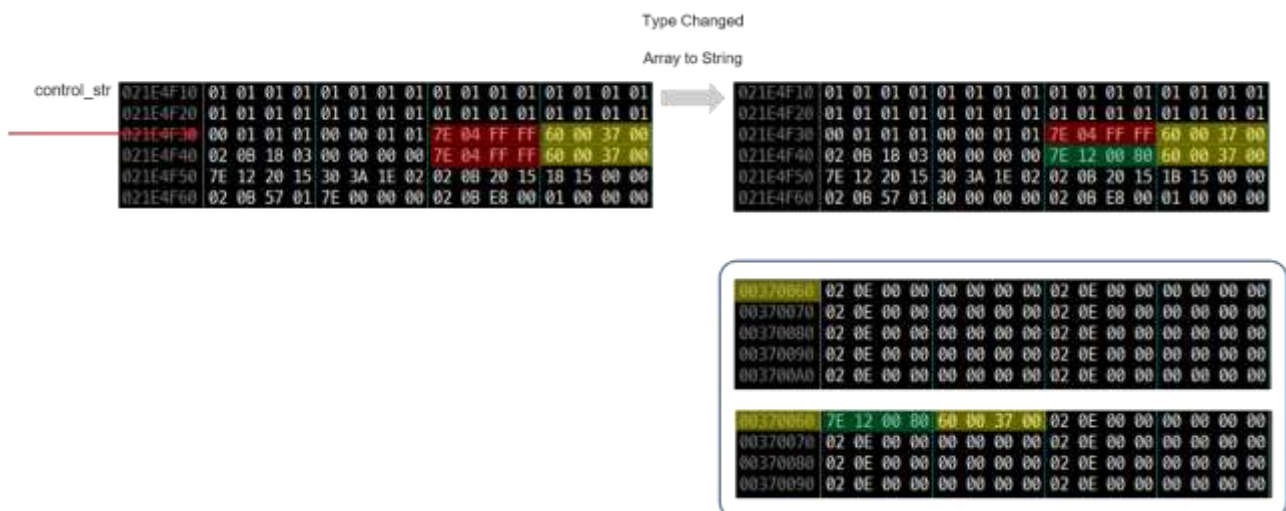
[그림 37] leaked_array 타입을 배열에서 문자열로 변환
