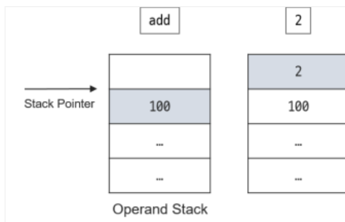
[그림 21] 피연산자 스택
