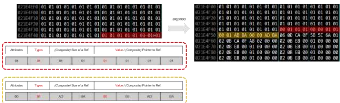
[그림 36] control_str 문자열이 변경
