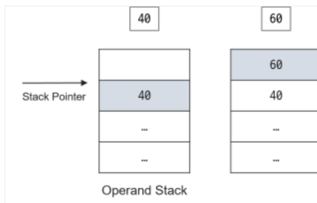
[그림 20] 피연산자 스택
