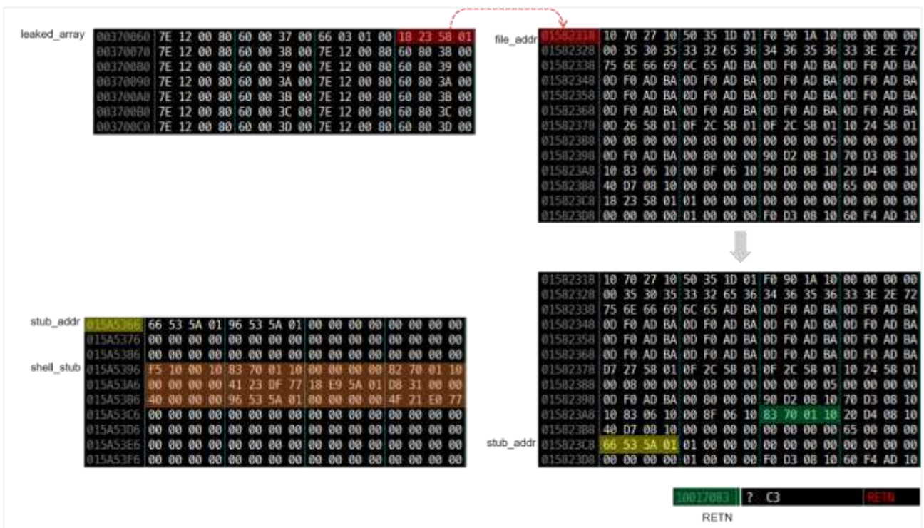
[그림 41] file_addr +B0 위치의 stub_addr와 +98 위치의 RETN 명령
