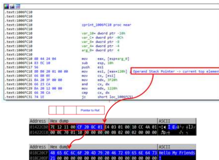
[그림 28] print 연산을 실행했을 때 피연산자 스택
