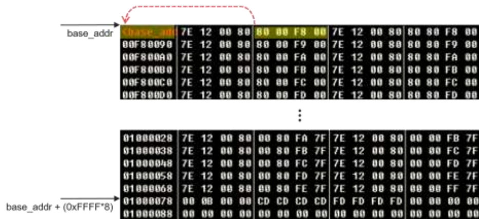
[그림 38] base_addr 주소를 이용하여 leaked_array 배열에 Element 추가
