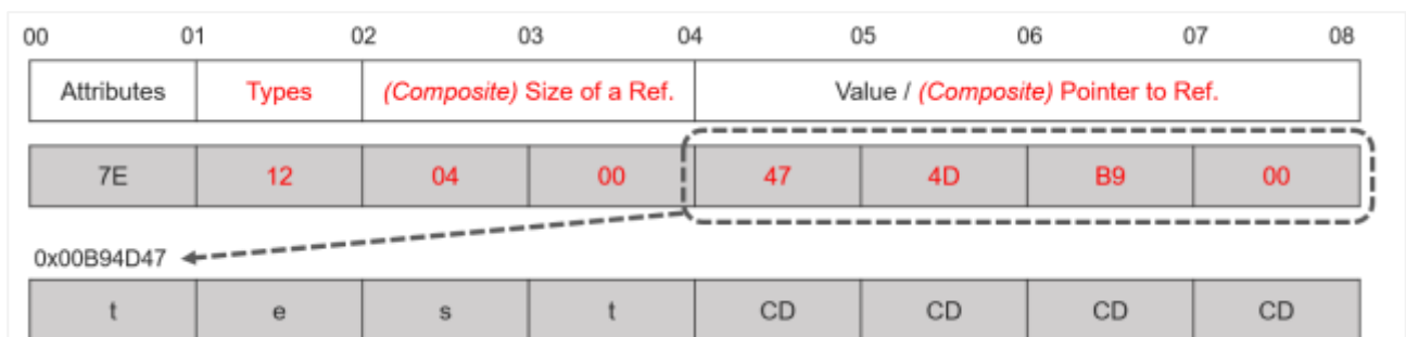
[그림 17] 메모리에 저장된 string 타입 객체
