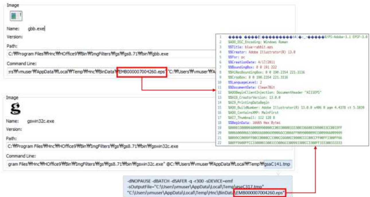
[그림 6] 고스트스크립트 프로세스(gbb.exe, gswin32c.exe)의 EPS 파일 접근
