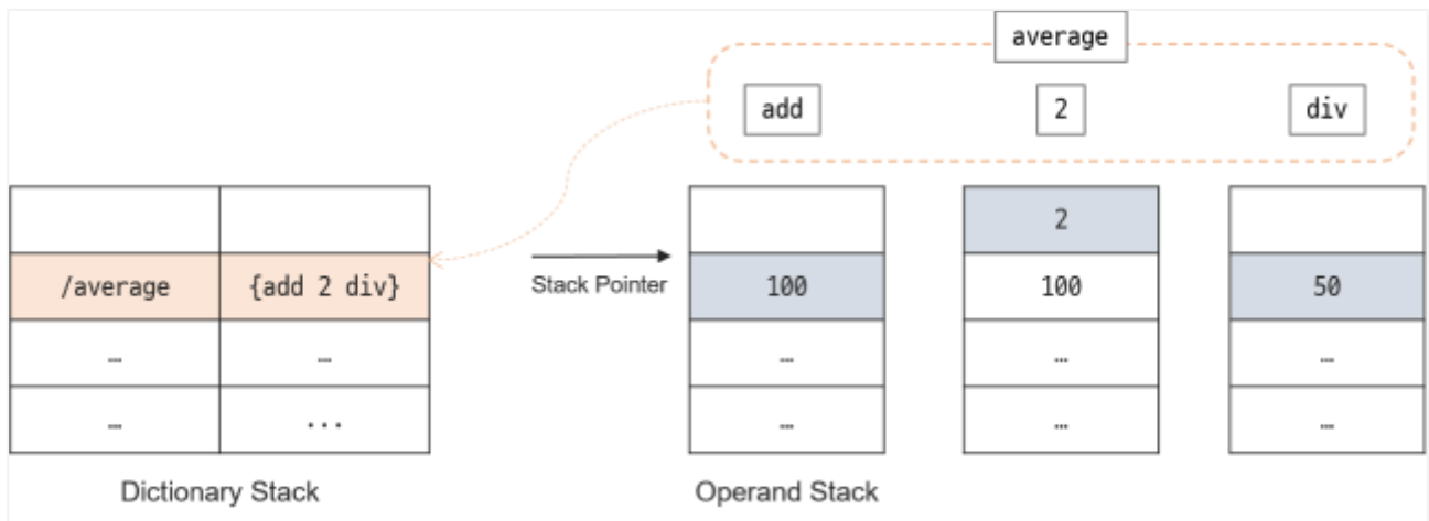
[그림 26] 딕셔너리 스택과 피연산자 스택
