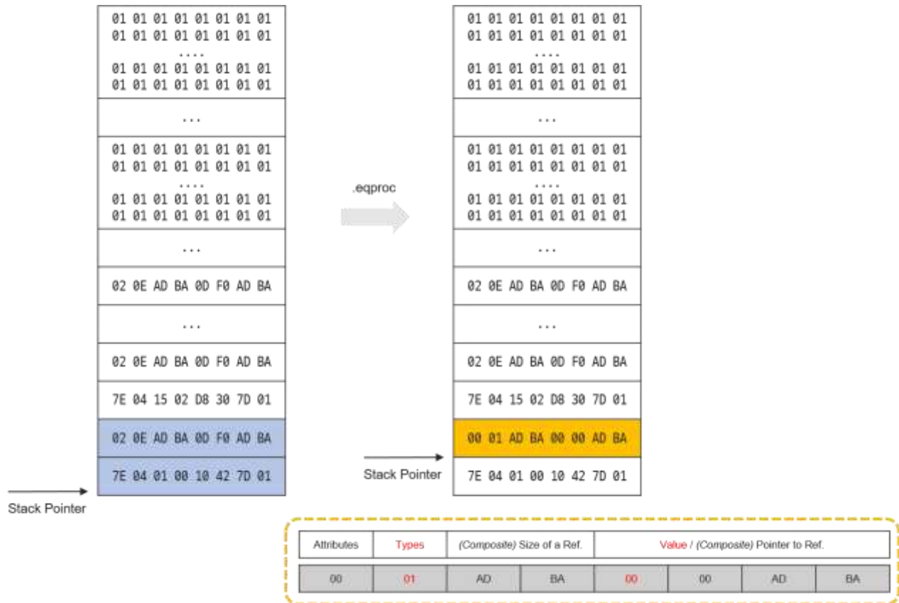
[그림 35] .eqproc 연산 이후의 스택 상태
