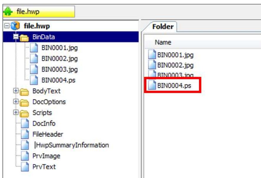
[그림 3] EPS 파일이 삽입된 한글 문서 파일 구조
