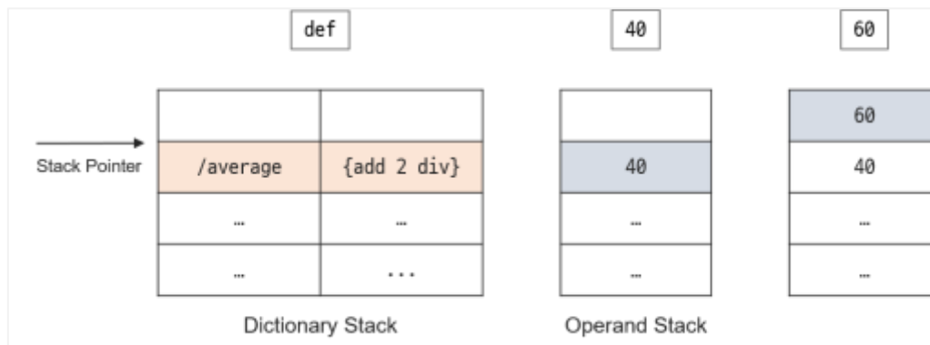
[그림 25] 딕셔너리 스택과 피연산자 스택
