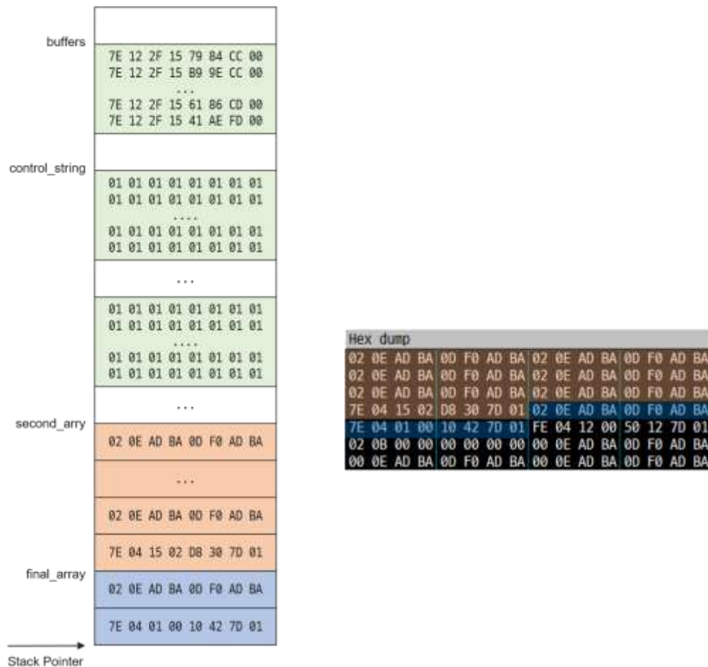
[그림 34] 스프레이 이후에 스택의 상태
